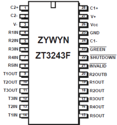
28-Pin SSOP/TSSOP/WSOIC
