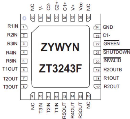
32-Pin VQFN
