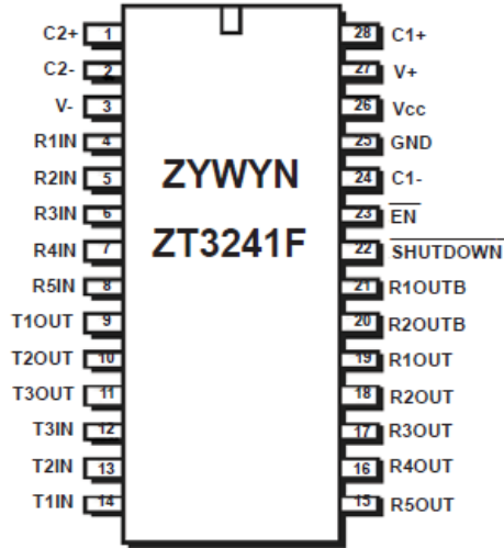
28-Pin SSOP/TSSOP/WSOIC
