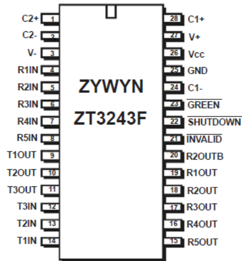
28-pin SSOP/TSSOP/WSOIC
